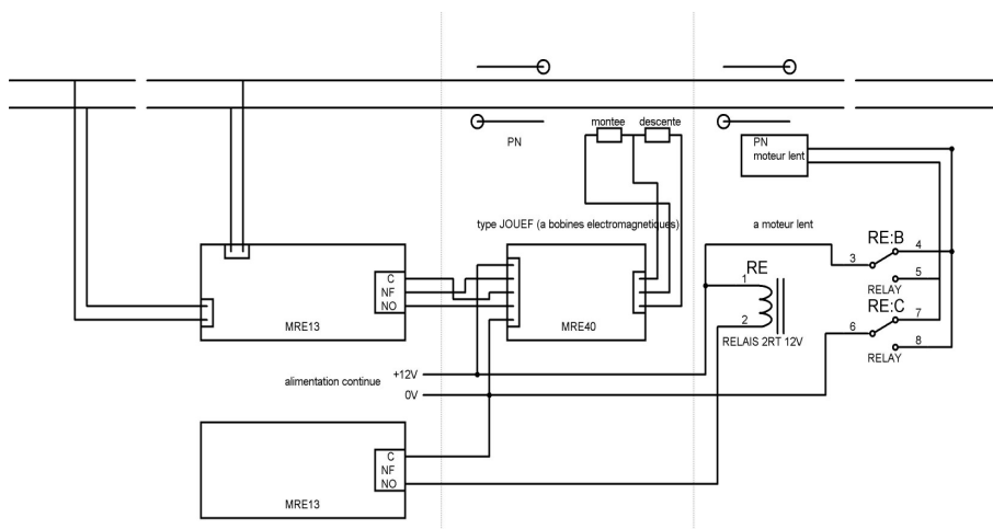
Automatisation d'un passage a niveau
